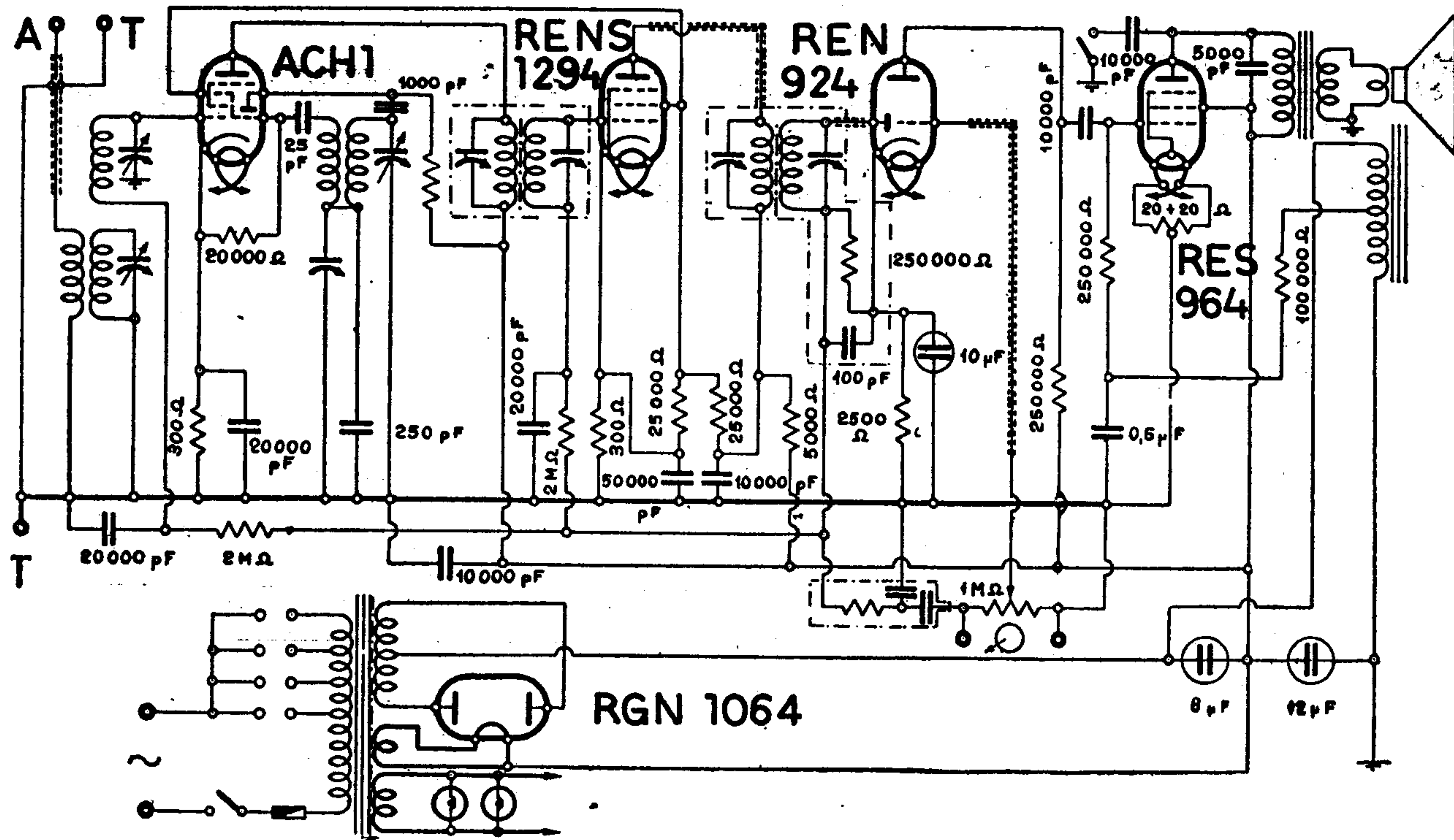
SIEMENS S. A. - MOD. « T 557 »
